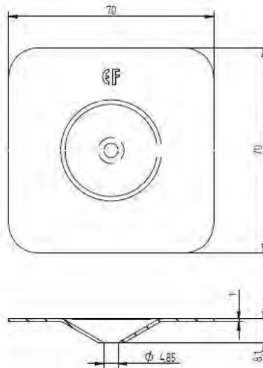
Eurofast DVP-EF-7070D
