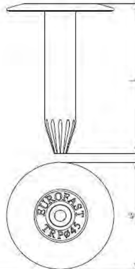
Eurofast TRP-45
