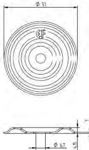
Eurofast DVP-EF-51N
