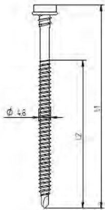
Eurofast EDS-BZTR 4,8 x L
