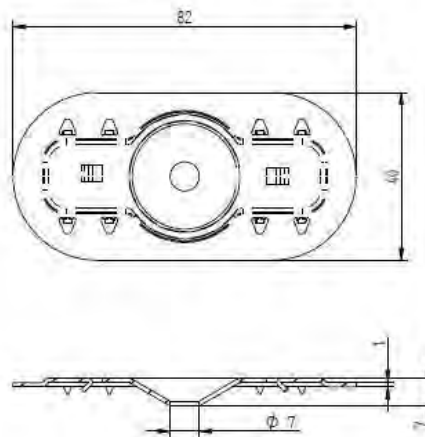
Eurofast DVP-DFB8240D
