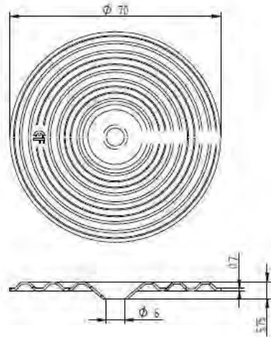
Eurofast DVP-EF-7007D
