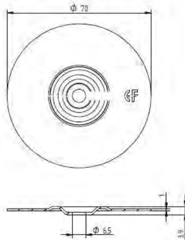
Eurofast DVP-EF-7010N
