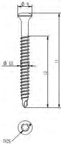
VRF Eurofast EDS-B 5,5
