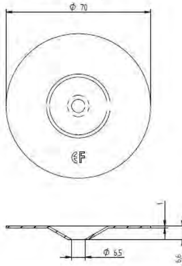
Eurofast DVP-EF-7010D
