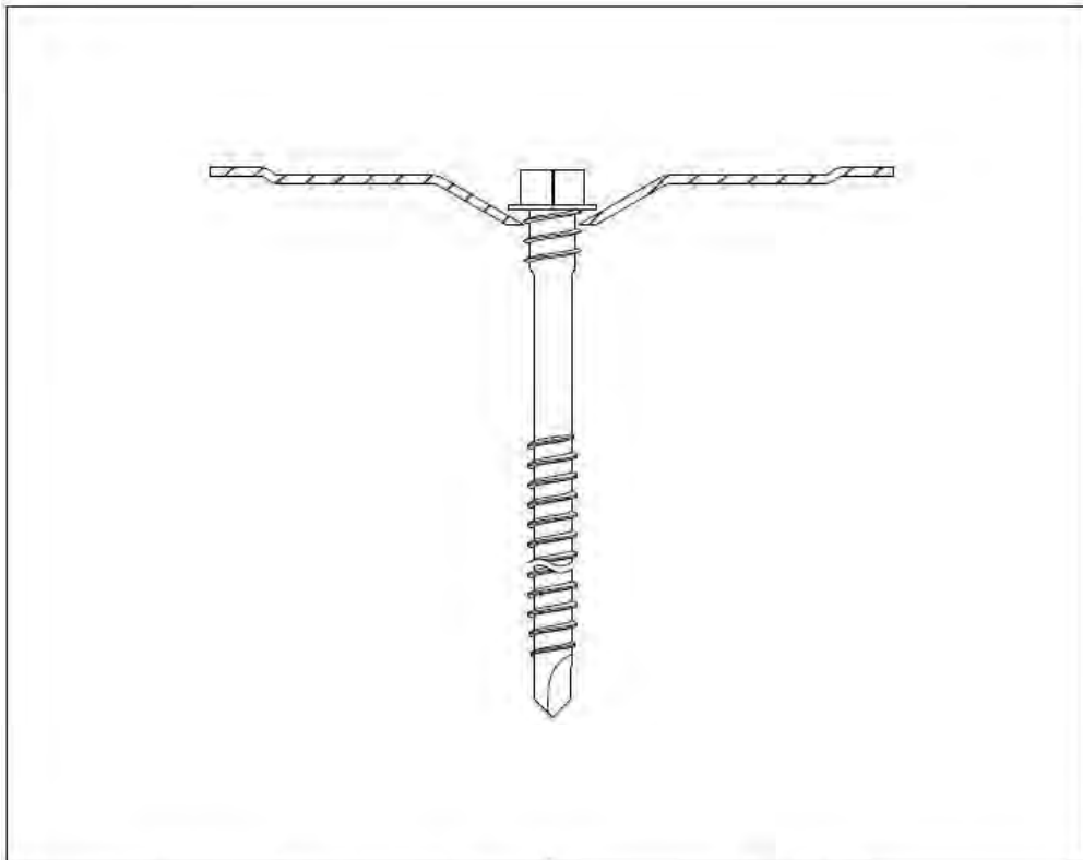
Eurofast DVP-EF-8040D
