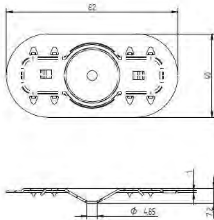
Eurofast DVP-EFB8240D
