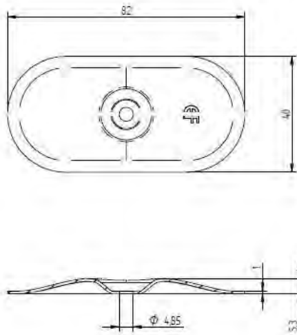
Eurofast DVP-EF-8240XH
