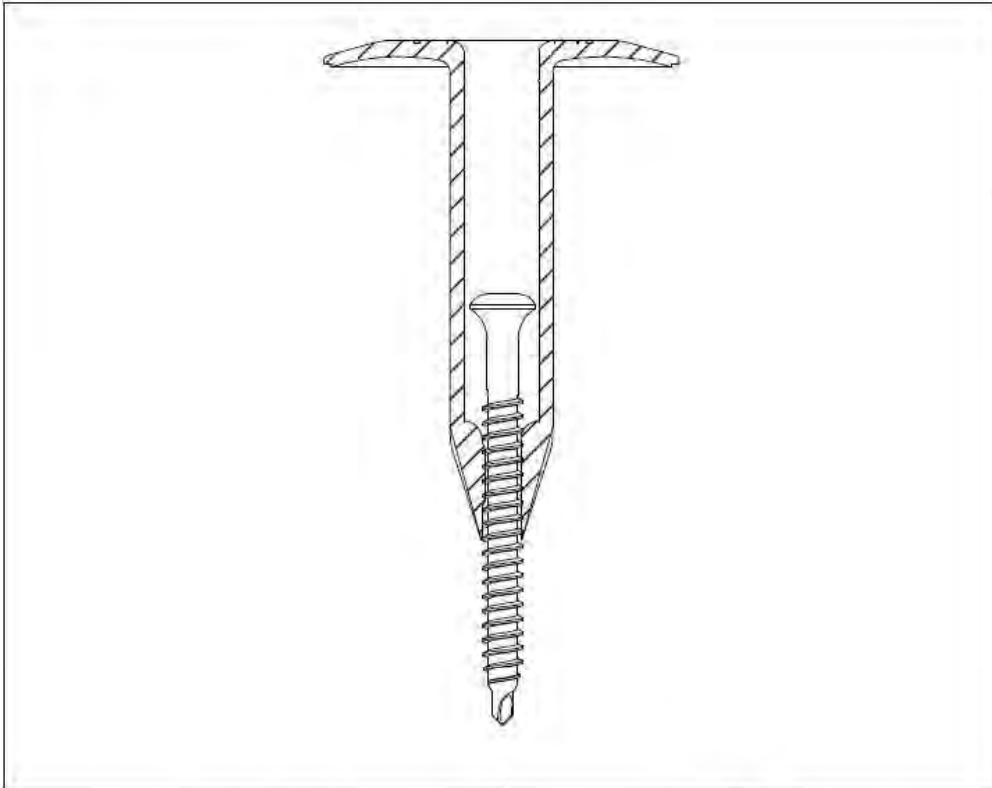
Eurofast TLK- 45
