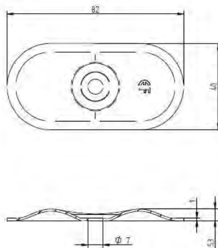
Eurofast DVP-DF8240XH
