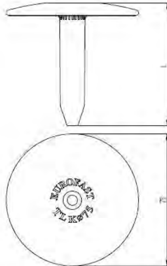
Eurofast TLK-75
