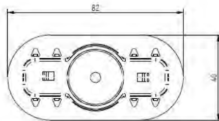
Eurofast DVP-EFB8240D
