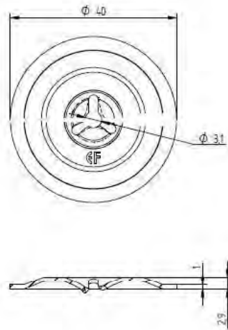
Eurofast DVP-EF-4010N3
