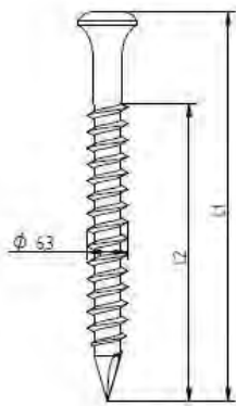
Eurofast EFHD 6,3 x L
