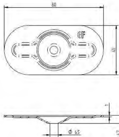
Eurofast DVP-EF-8040D
