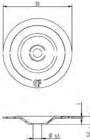
Eurofast DVP-EF-5010D
