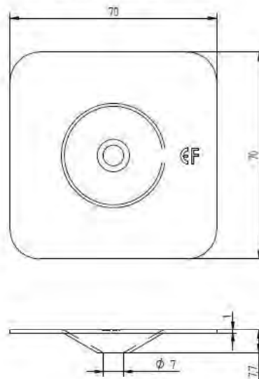
Eurofast DVP-DF-7070D
