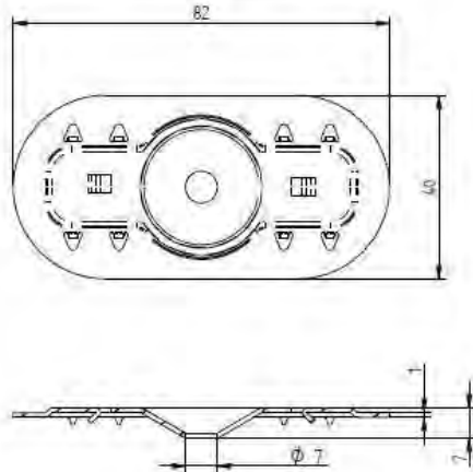
Eurofast DVP-DFB8240D
