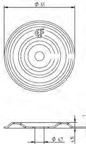
Eurofast DVP-EF-51N
