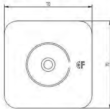
Eurofast DVP-DF-7070D
