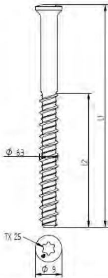
Eurofast EFR 6,3 x L
