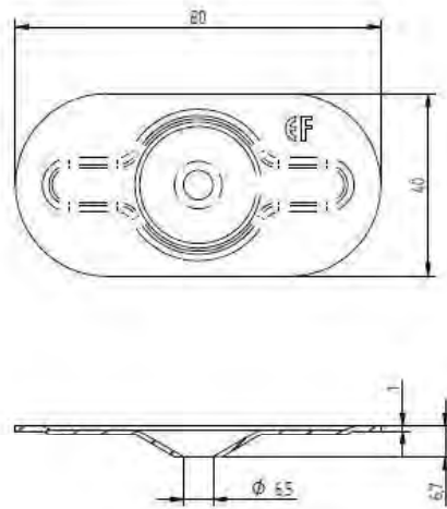
Eurofast DVP-EF-8040D
