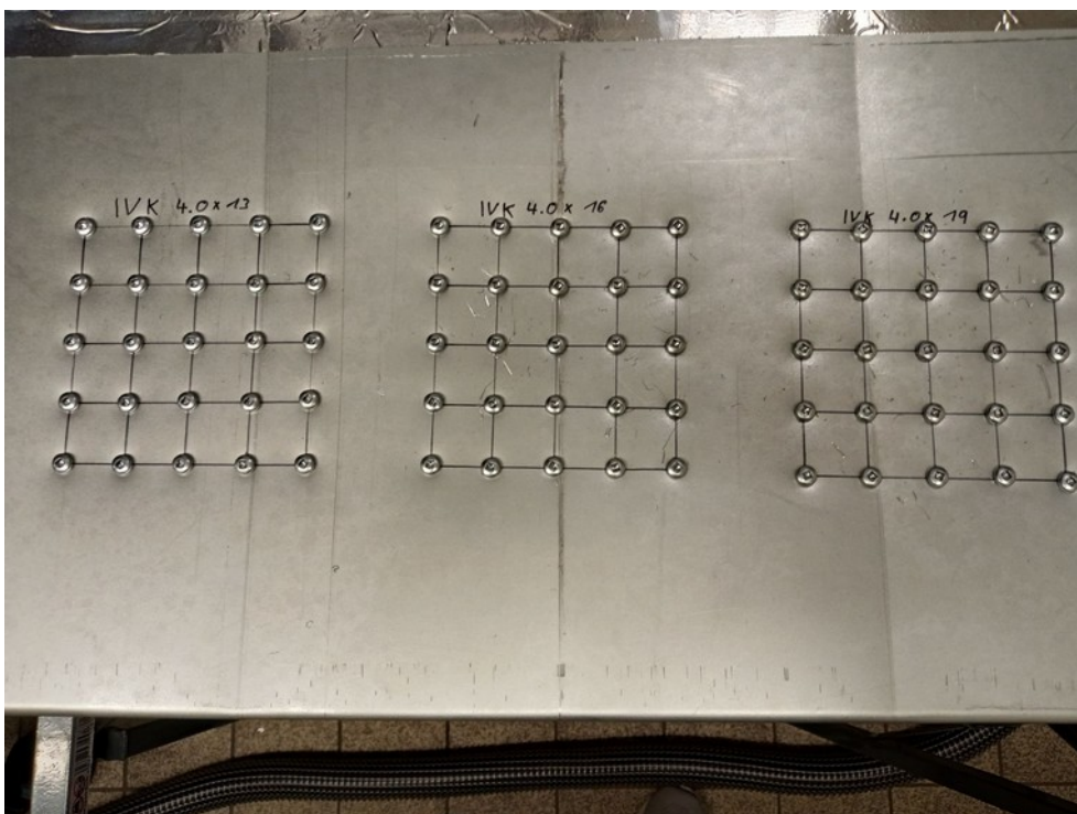
Abbildung 4.4: Luftkanal mit 75 Dünnschraube, je 25 x 4KT-GR2-4,0X13, 25 x 4KT-GR2-4,0X16 und 25 x 4KT-GR2-4,0X19
