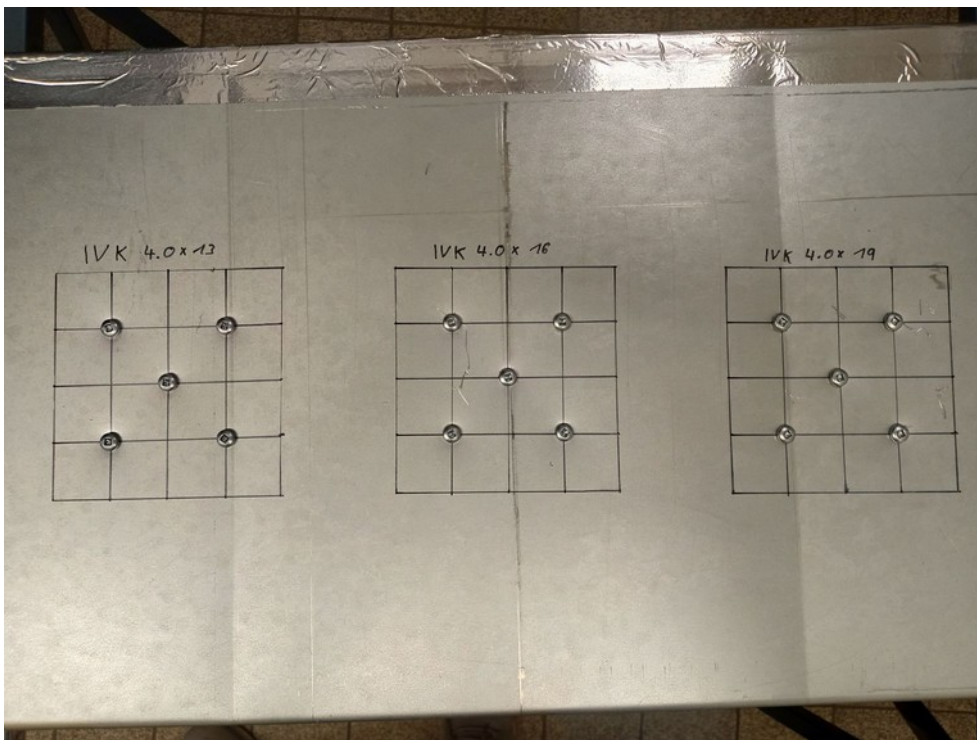
Abbildung 4.3: Luftkanal mit 15 Dünnschraube, je 5 x 4KT-GR2-4,0X13, 5 x 4KT-GR2-4,0X16 und 5 x 4KT-GR2-4,0X19
