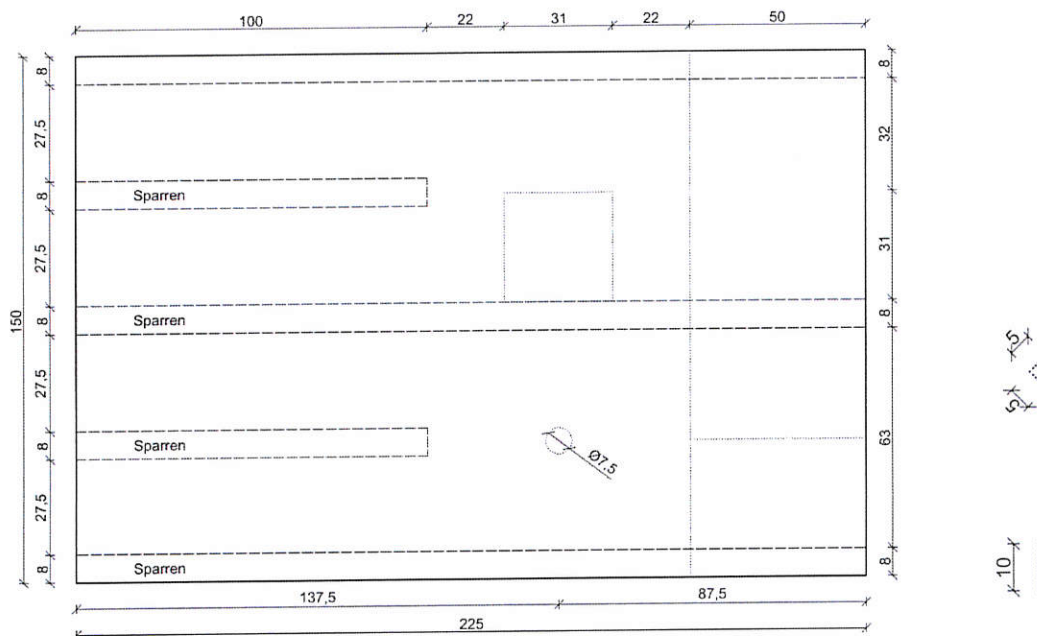
Abbildung 1: Prüfkörper zur Prüfung der erhöhten Regensicherheit bei Dachneigungen < 5^\circ , Draufsicht, rechts Detail der Verletzungen der Folie
